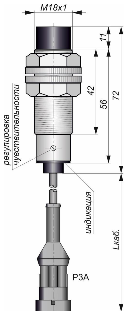
Габаритный чертеж
