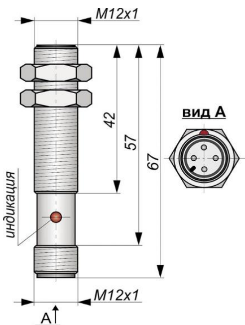
Габаритный чертеж
