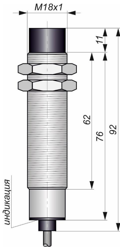
Габаритный чертеж
