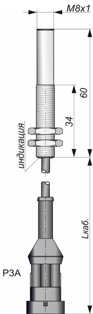
Габаритный чертеж
